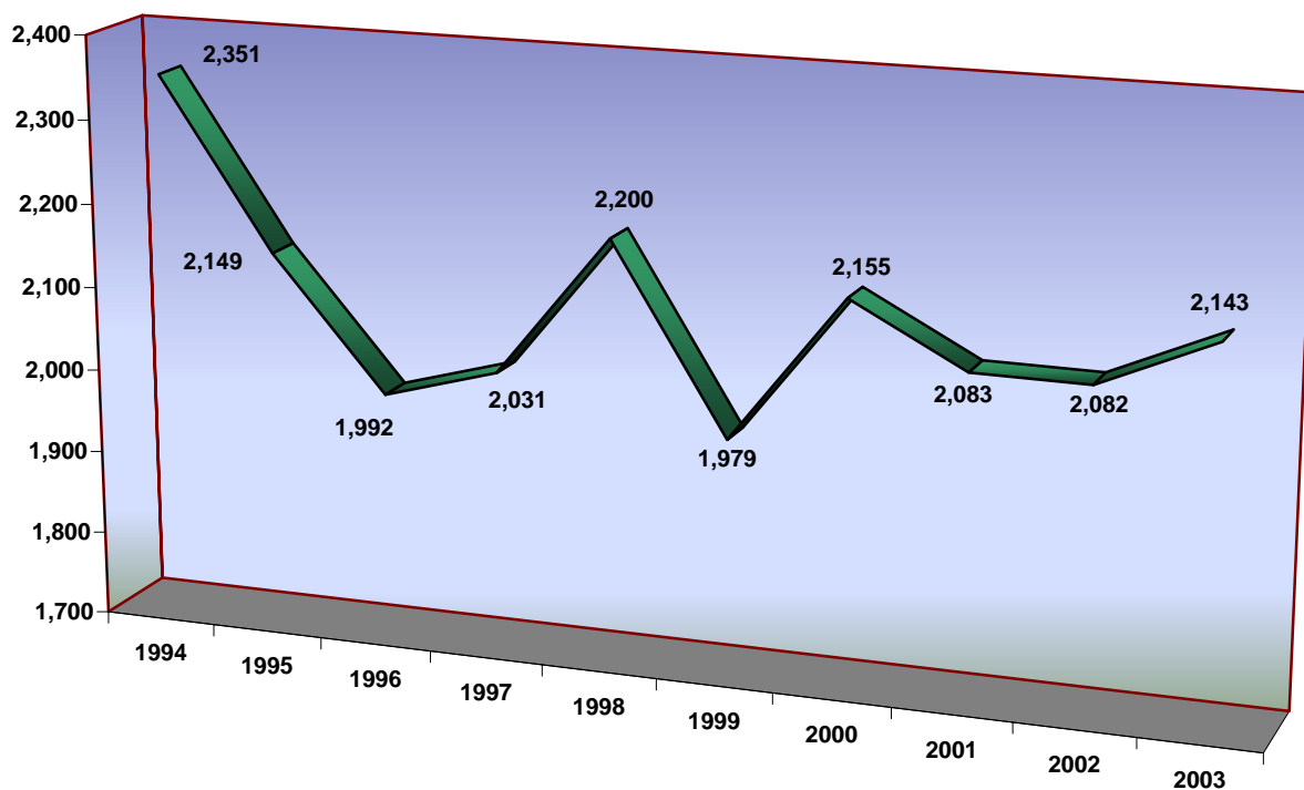
Arson Trend 1994 - 2003
